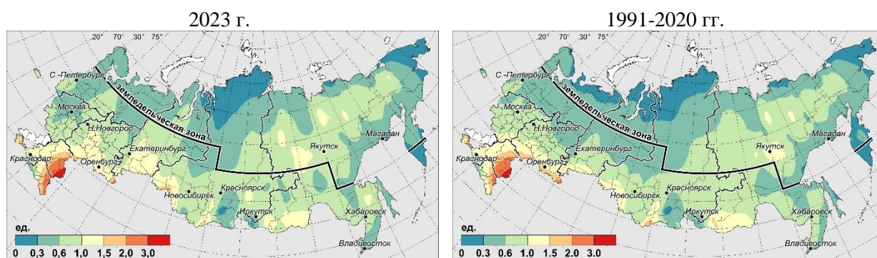
Рисунок 8.2 – Индекс сухости М.И. Будко за 2023 год и средние значения за 1991–2020 гг.
