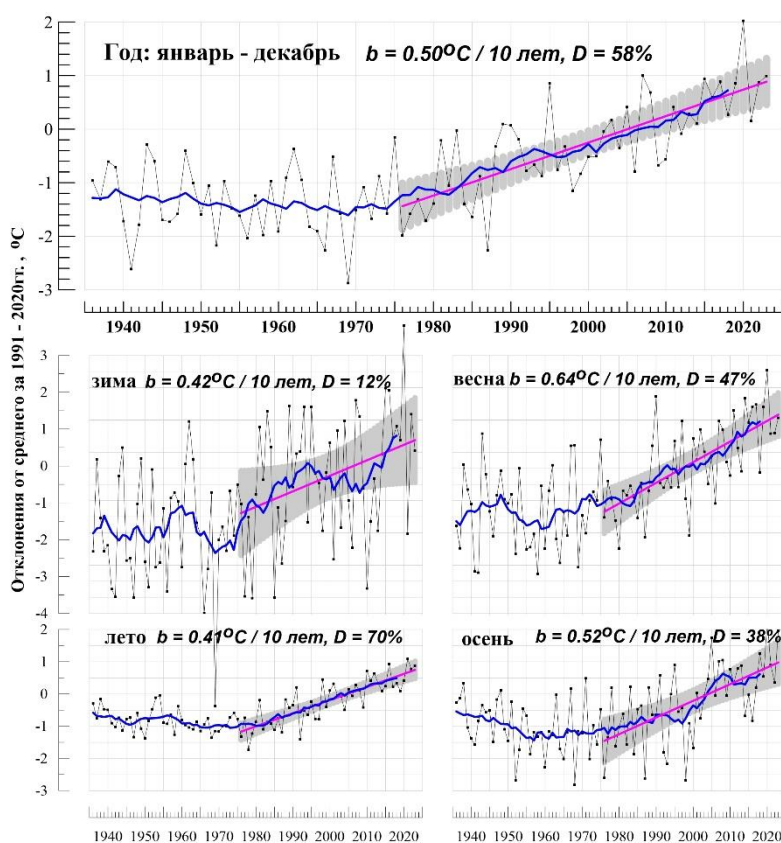
Рисунок 1.1 – Средние годовые (вверху) и сезонные аномалии температуры приземного воздуха (°C), осредненные по территории России, 1936-2023 гг.
